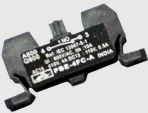
PBE-4FC-A (1NO)
